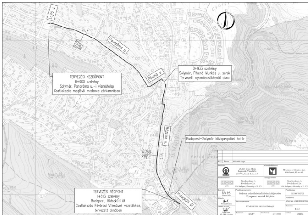
A vezeték solymári szakasza 1813 méter hosszú, 250 mm átmérőjű KPE csővekből áll.
